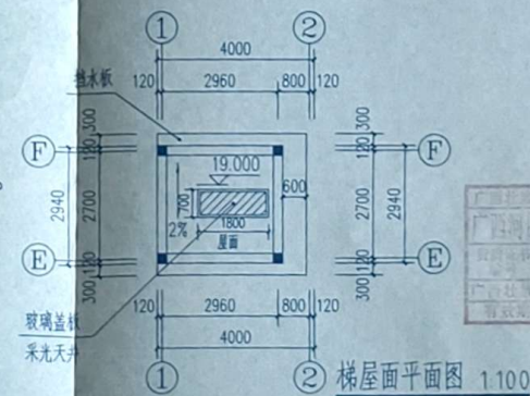
屋面平面图 1:100
