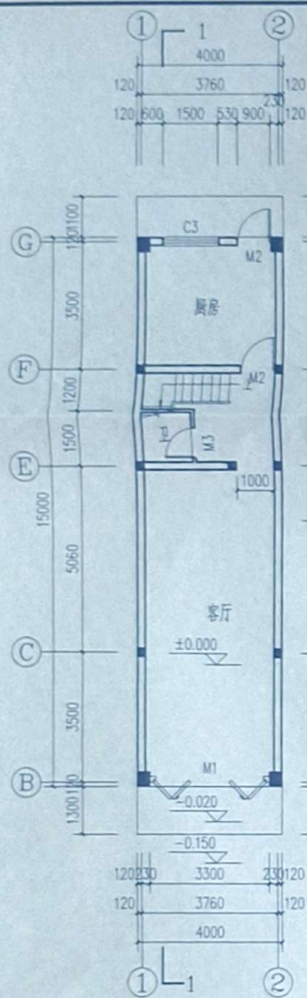
一层平面图 1:100
