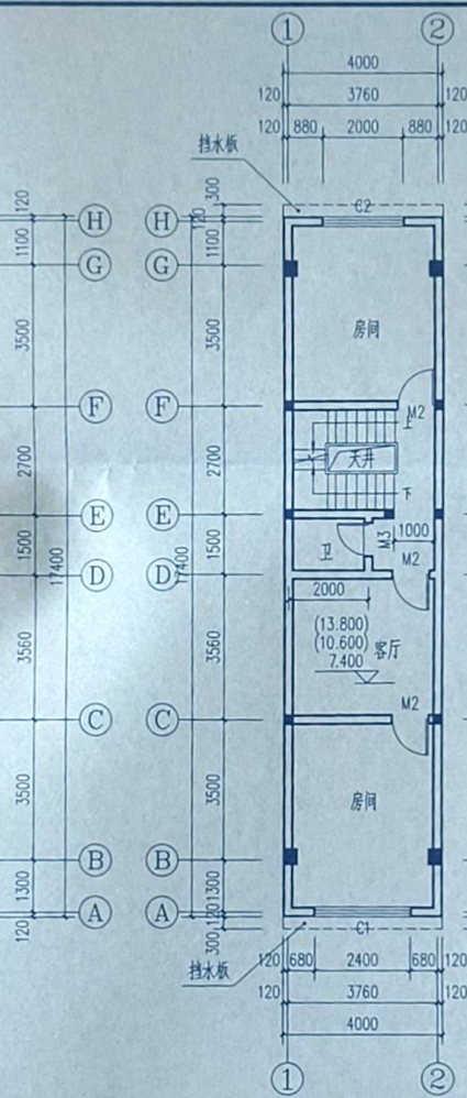
三~五层平面图 1:100
