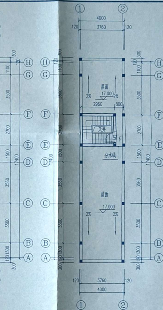
屋面平面图 1:100
