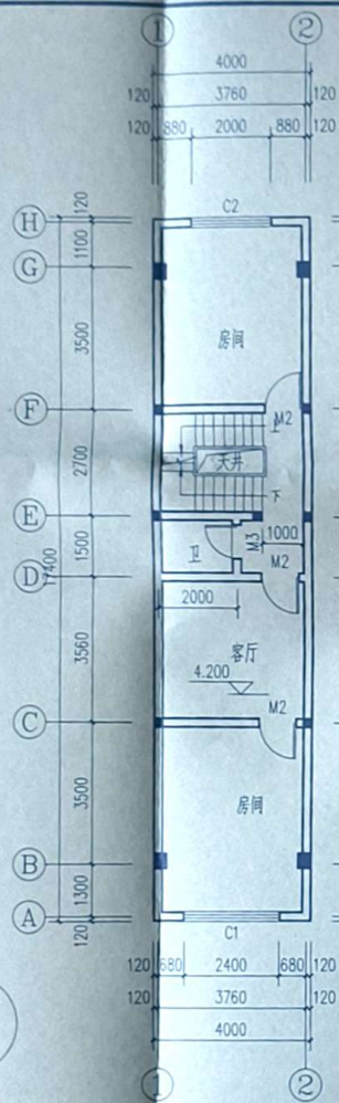
二层平面图 1:100
