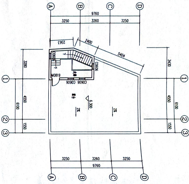
屋面平面图 1:100
