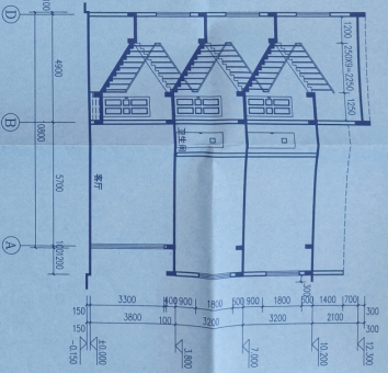
1-1剖面图 1:100
